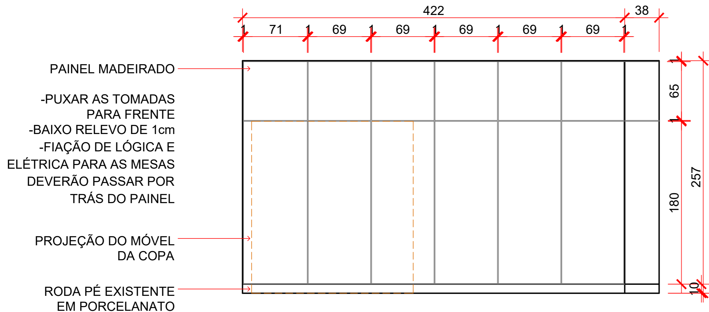
VISTA 3- PAINEL Esc 1/25
