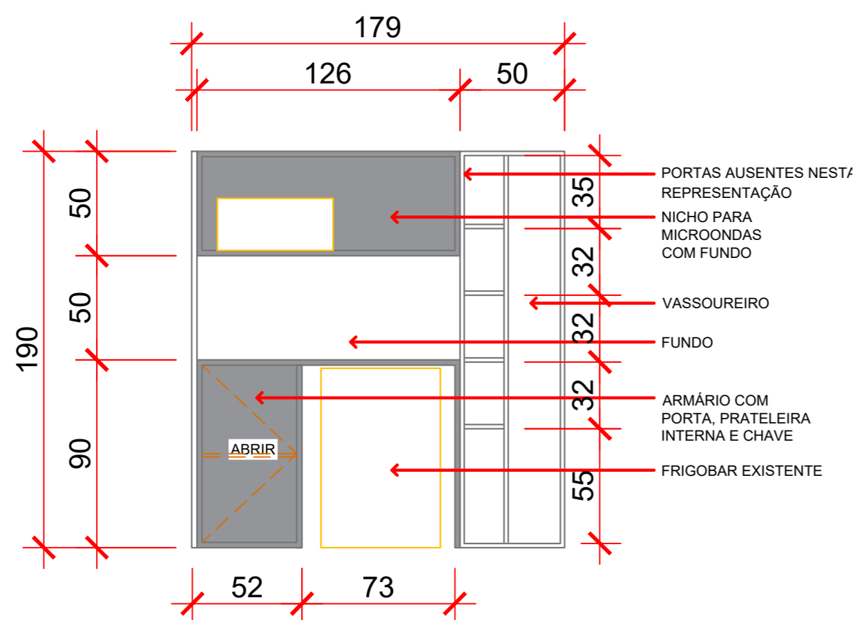
VISTA MÓVEL COPA Esc 1/25
